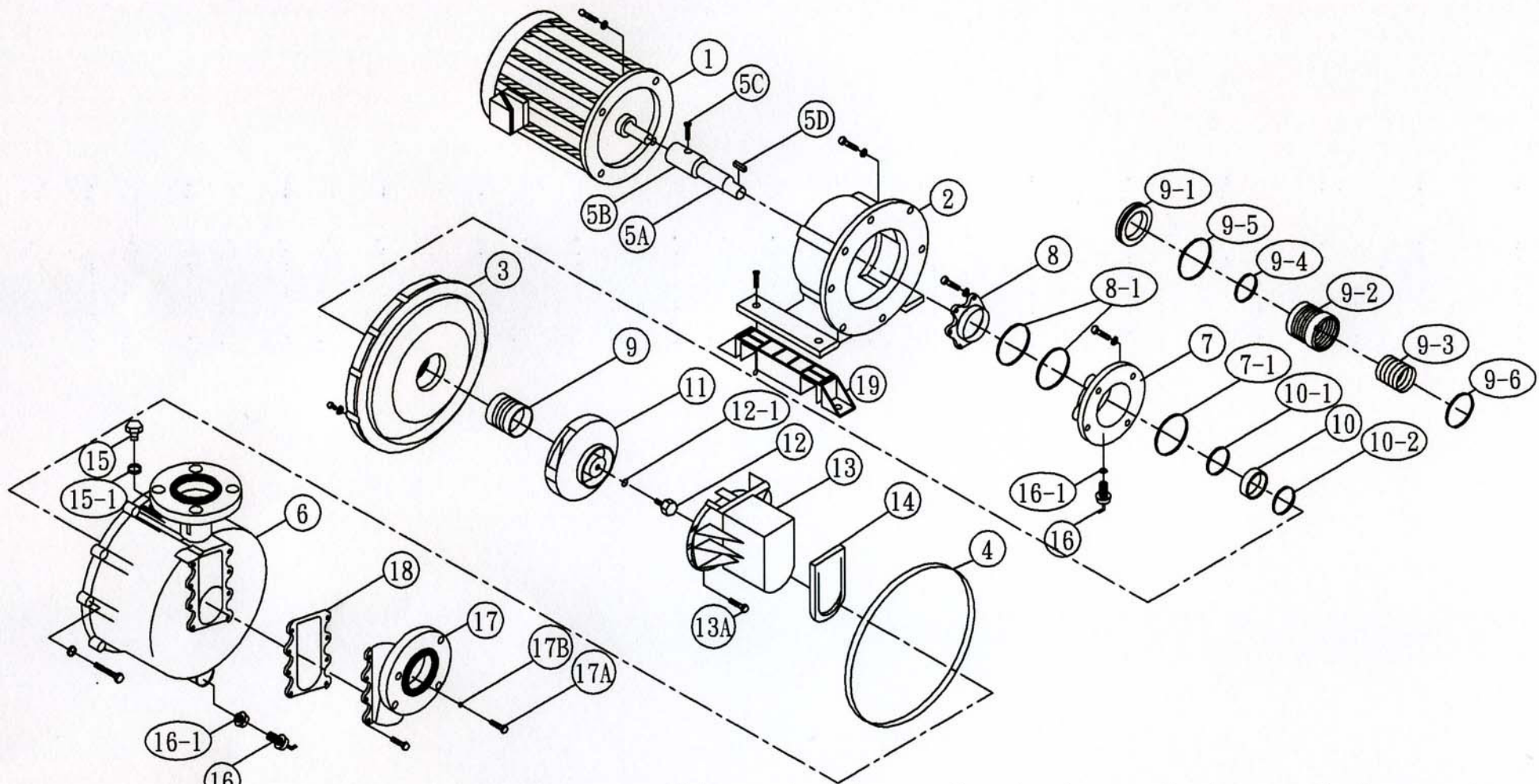
GD 同軸自吸式耐酸鹼泵浦立體系統圖
